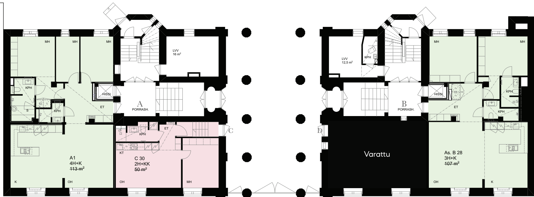
GRAND HORIZON Pinnatelli & Kauri Alustava 03/2022
