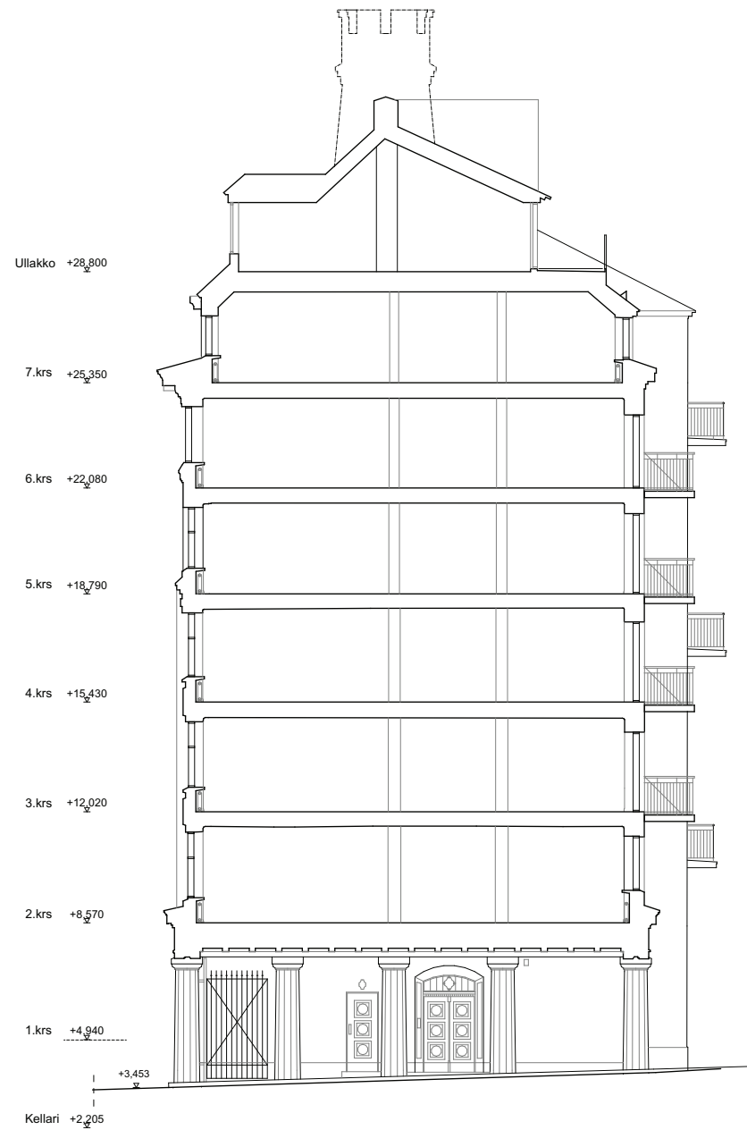
GRAND HORIZON Periaateleikkaus Alustava 03/2022
